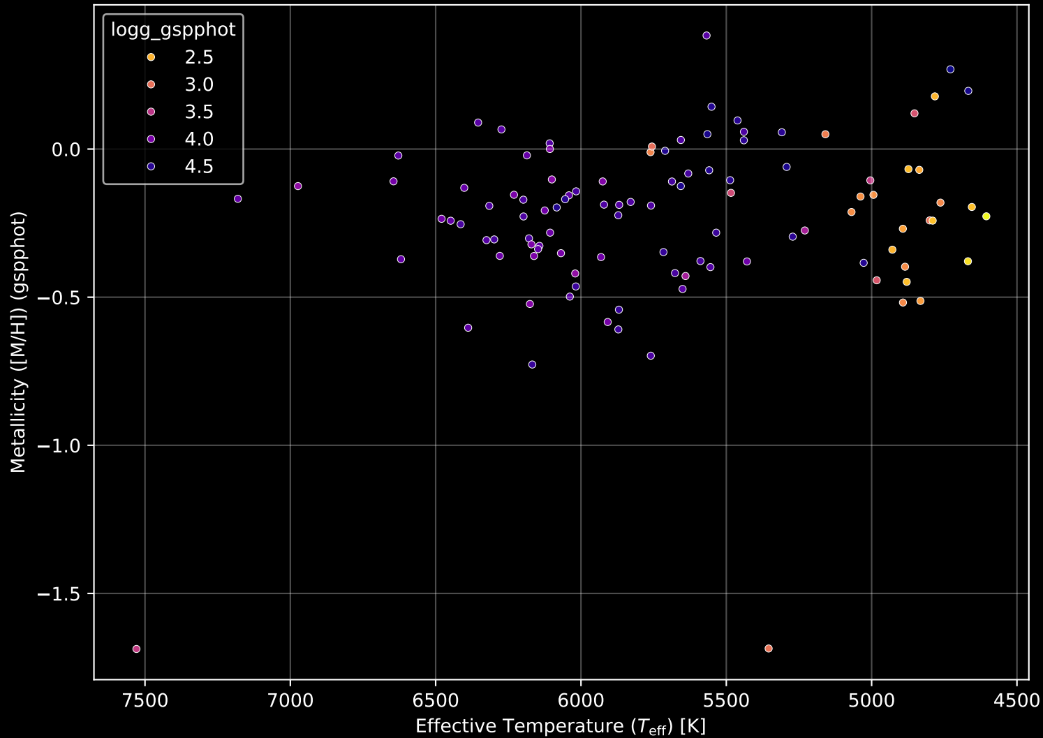
GALAH DR4 Field: [7213] Stellar Population Parameters (n= 106)
